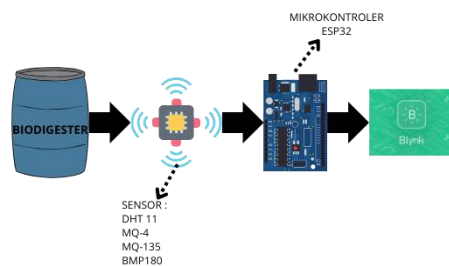
GAMBAR 1. Sistem Kerja Alat
