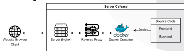
GAMBAR 2 (Server Arsitektur Diagram)
