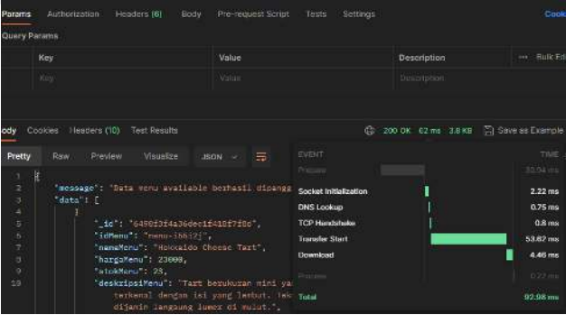
GAMBAR 5 (Performa Get data available menu: 62ms – pelanggan)
