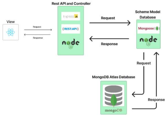
GAMBAR 1 (Diagram Arsitektur Cafeasy)
