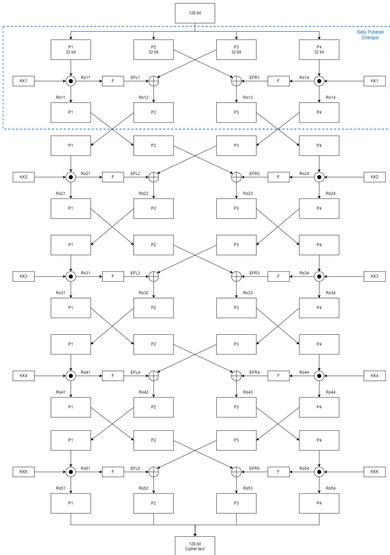
GAMBAR 5 Proses enkripsi
