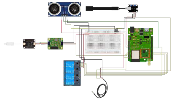
Gambar 4 Skematik Alat AWNDES
