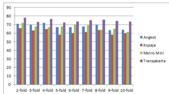
Gambar 4-1 Grafik akurasi cross validation
