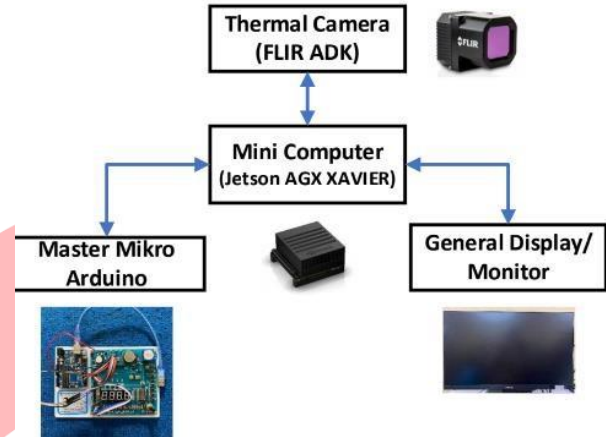
GAMBAR 7 Konstruksi Hardware
