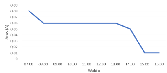
GAMBAR 12. Arus Yang Diberikan Modul Sel Surya
