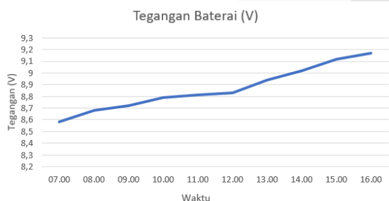
Gambar 10. Hasil Pengisian Baterai Menggunakan Modul Sel Surya
