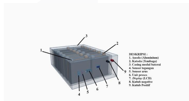
GAMBAR 2. Desain Sistem Baterai Aluminium
