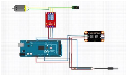
Gambar 7 Perancang Aerator
