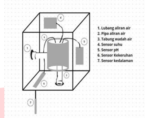
GAMBAR 1. Desain sistem
