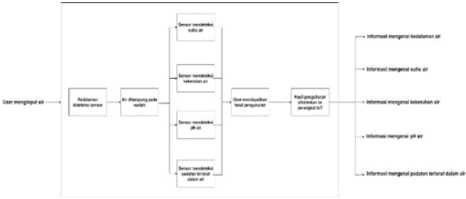
GAMBAR 3 Function tree Sistem Monitoring dan Klasifikasi Polusi Air Sungai
