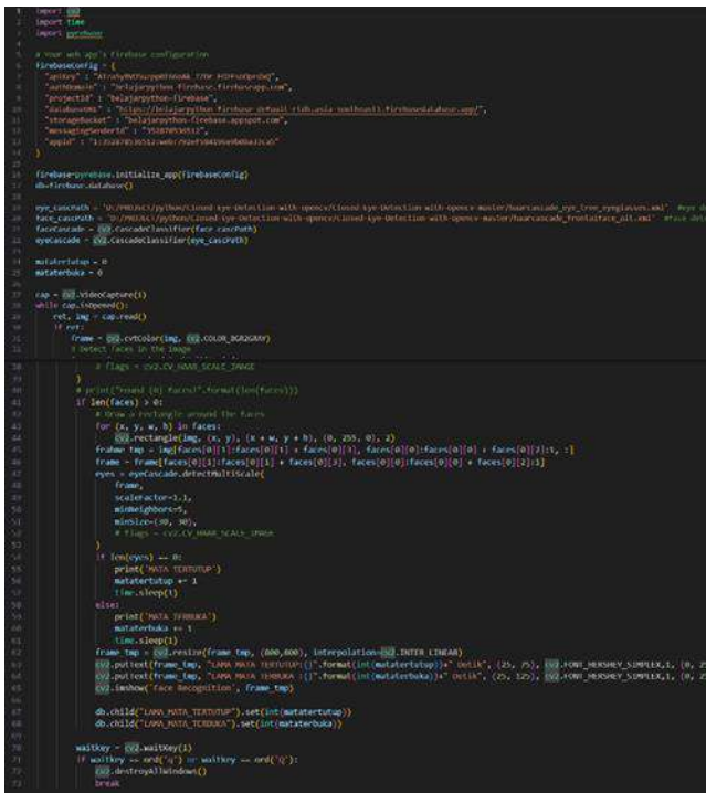
GAMBAR 3.3 Source code untuk penangkapan citra mata
