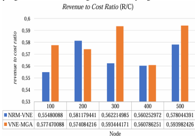
GAMBAR 4.3 SKENARIO REVENUE TO COST RATIO (R/C) PADA METODE NRM-VNE DAN VNE-MGA
