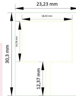
GAMBAR 3.3 DESAIN AWAL ANTENA
