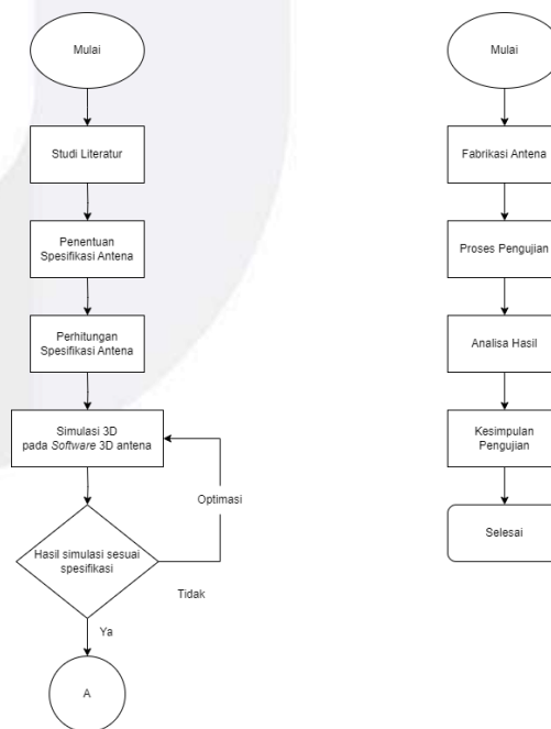
GAMBAR 3.2 DIAGRAM ALIR SISTEM
