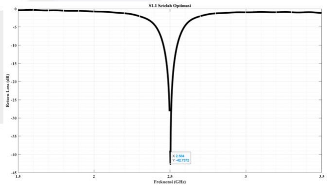
GAMBAR 4.5 RETURN LOSS SETELAH OPTIMASI
