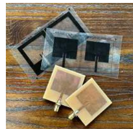
GAMBAR 3.5 ANTENA REALISASI
