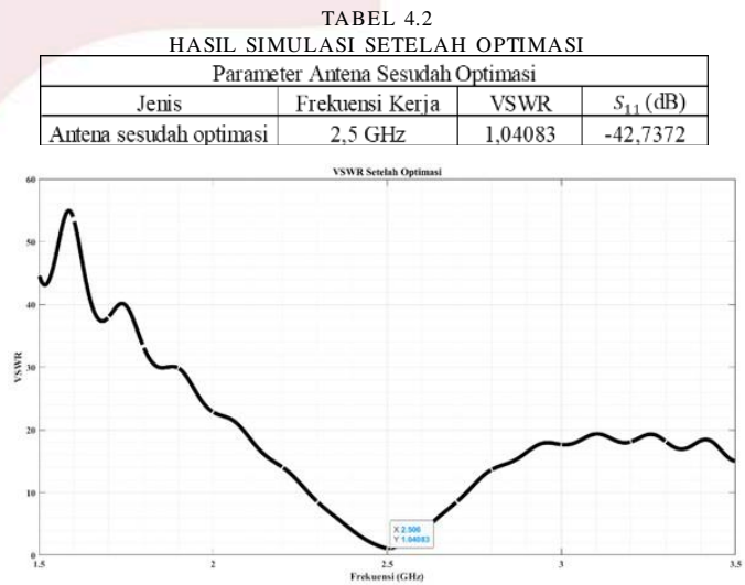
Gambar 4.4 VSWR Setelah Optimasi
