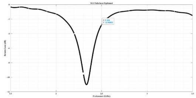
GAMBAR 4.2 RETURN LOSS SEBELUM OPTIMASI
