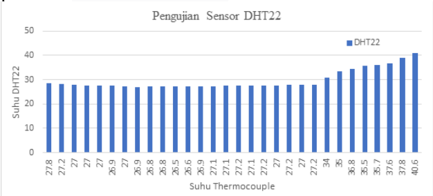
GAMBAR 4 Grafik Perbandingan Sensor Dht22
