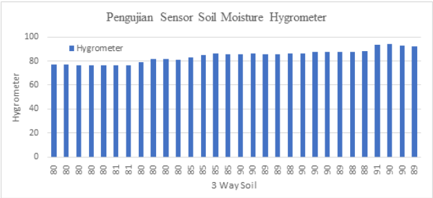
GAMBAR 5 Hasil Pengujian Sensor Hygrometer
