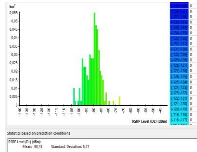
GAMBAR 10a: Rsrp Awal
