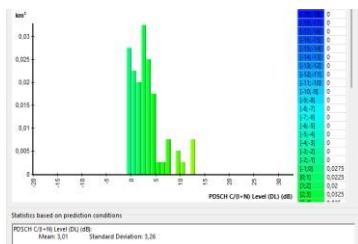
GAMBAR 9a: SINR Awal
