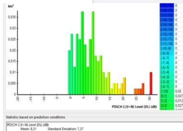
GAMBAR 9b: SINR Optimasi
