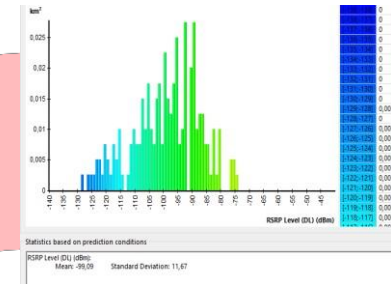
GAMBAR 10b: RSRP Optimasi
