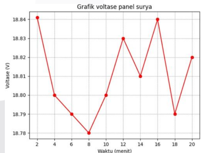
GAMBAR 8. Grafik Pengukuran Tegangan Panel Surya
