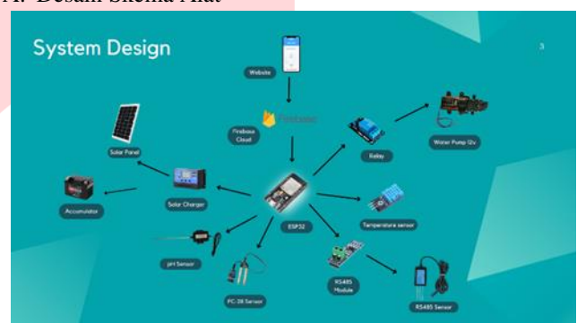
Gambar 1. Desain Skema Alat
