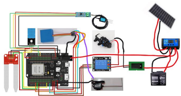
GAMBAR 4. Schematic Desain Perangkat Penyirama
