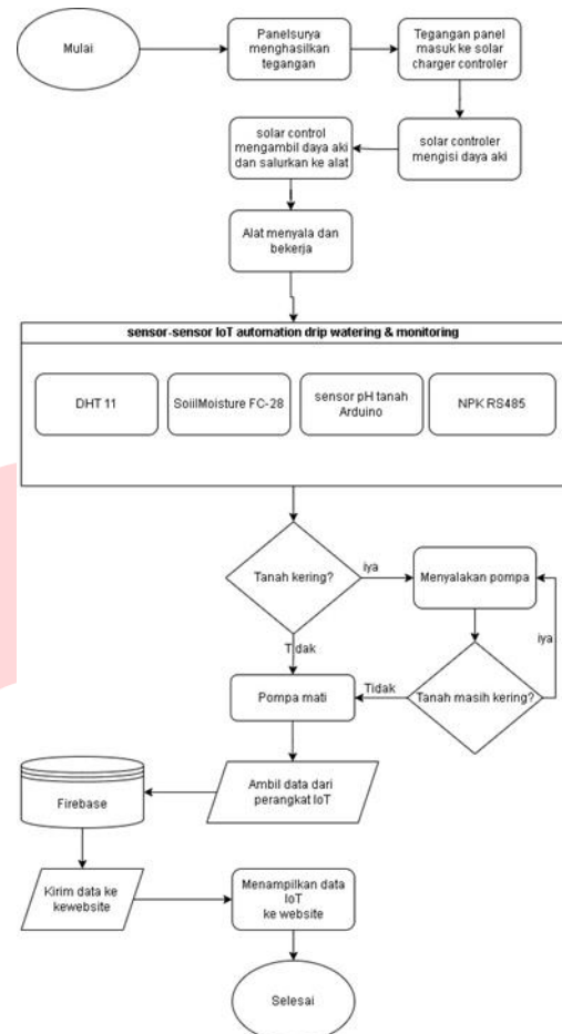
GAMBAR 3. Diagram Alur Sistem Pemantauan dan Penyiraman
