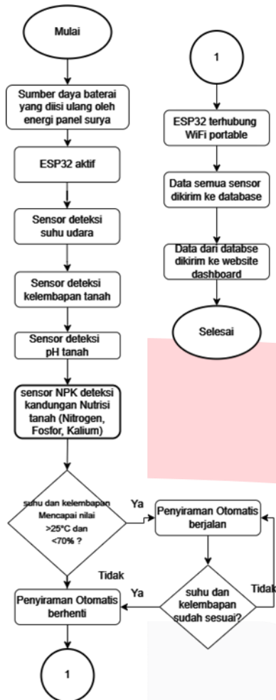
GAMBAR 2. Diagram Alur Penyiraman
