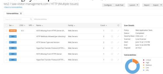
GAMBAR 13 Hasil Pengujian dengan Nessus Essentials
