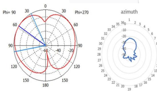
GAMBAR 4 Polarisasi azimuth antenna dengan metasurface
