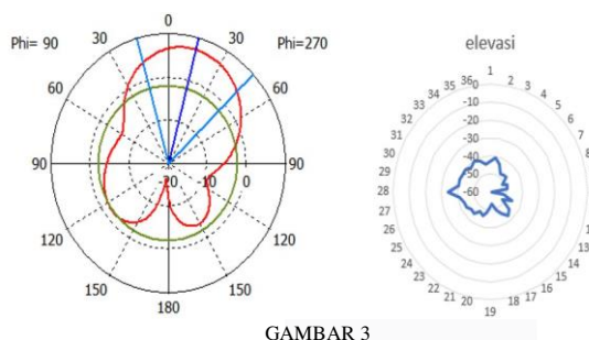
GAMBAR 3 Polarisasi elevasi antenna dengan metasurface
