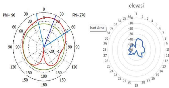
GAMBAR 1 Polarisasi elevasi antenna
