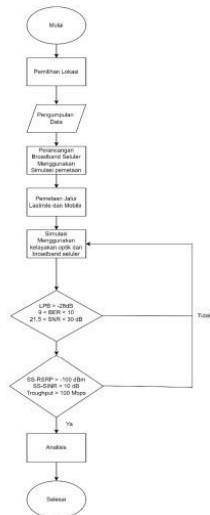
GAMBAR 1. Flowchart Perencanaan Lastmile dan FTTM
