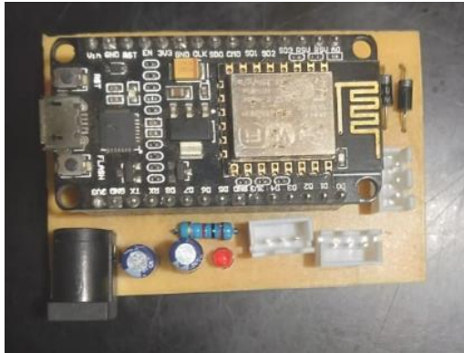
GAMBAR 7 (Implementasi Alat)
