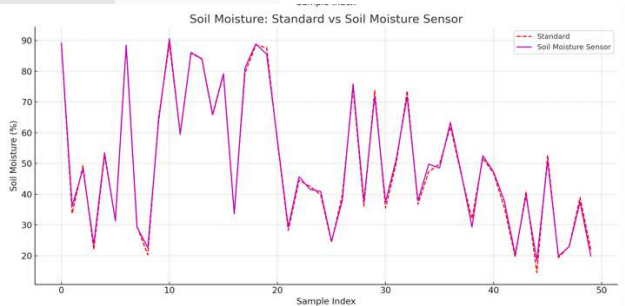
GAMBAR 11 (Grafik akurasi Soil Moisture)
