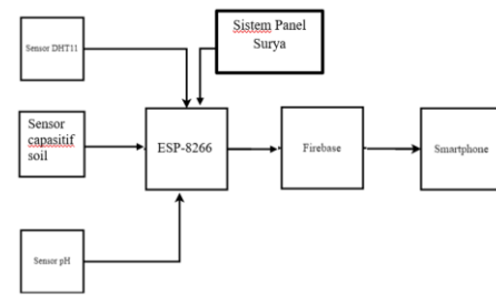
GAMBAR 1 (Blok Sistem)
