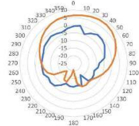
GAMBAR 21. Polaradiasi Elevasi Perban 3.5GHz
