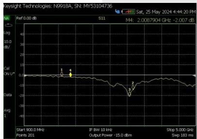
GAMBAR 6. S11 Perban 3.5GHz
