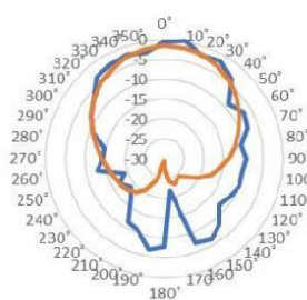
GAMBAR 24. Polaradiasi Azimuth Katun 3.5GHz
