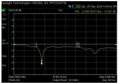
GAMBAR 8. S11 Perban 1.8GHz
