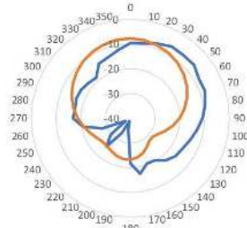
GAMBAR 22. Polaradiasi Azimuth Perban 1.8GHz
