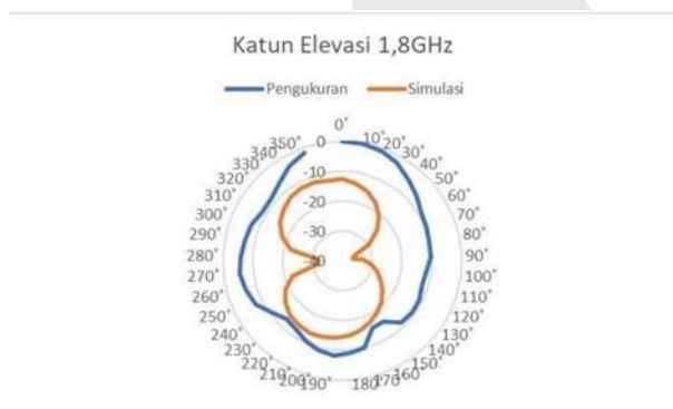
GAMBAR 27. Polaradiasi Elevasi Katun 1.8GHz
