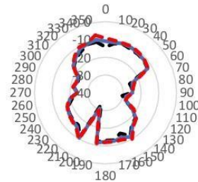
GAMBAR 19. Polarisasi Katun 1.8GHz
