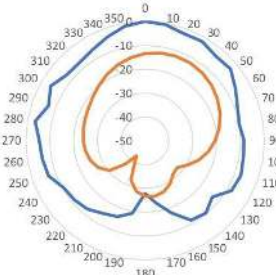
GAMBAR 23. Polaradiasi Elevasi Perban 1.8GHz
