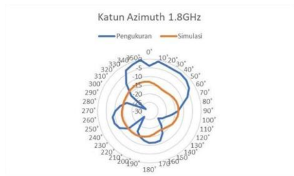
GAMBAR 26. Polaradiasi Azimuth Katun 1.8GHz
