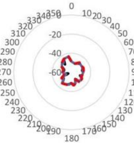
GAMBAR 17. Polarisasi Perban 1.8GHz
