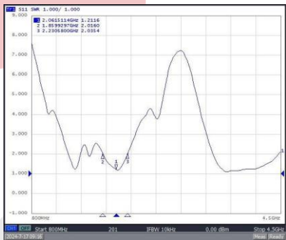
GAMBAR 9. VSWR Perban 1.8GHz
