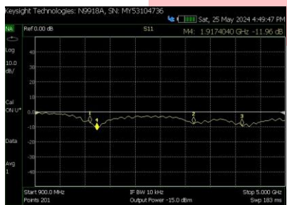
GAMBAR 12. S11 Katun 1.8GHz
