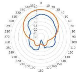
GAMBAR 20. Polaradiasi Azimuth Perban 3.5GHz
