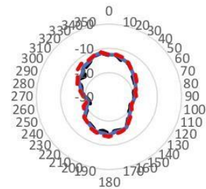
GAMBAR 18. Polarisasi Katun 3.5GHz
