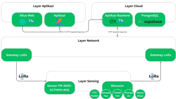
GAMBAR 3 Arsitektur Sistem Dicompos
