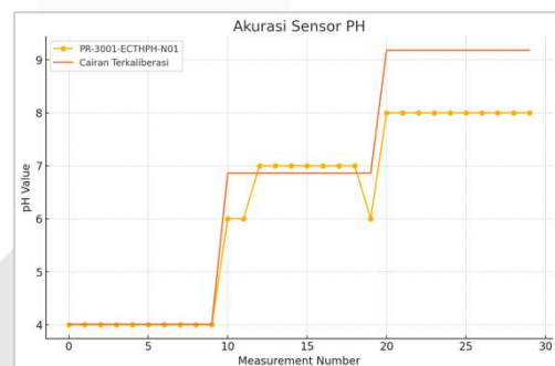
GAMBAR 11 Grafik Komparasi Akurasi Pengukuran pH
