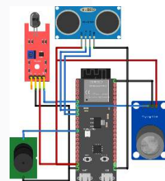
GAMBAR 3 (Contoh skematik alat)
