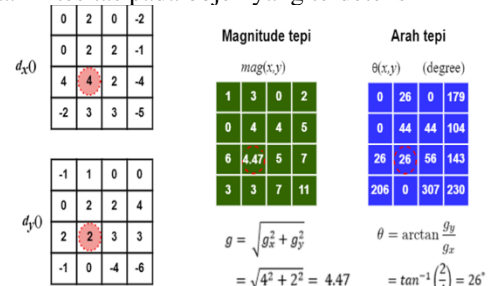
GAMBAR 4 contoh perhitungan HOG
