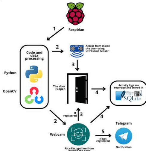
GAMBAR 1 Desain sistem
