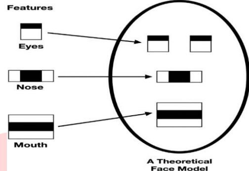
GAMBAR 3 Fitur Haarcascad
