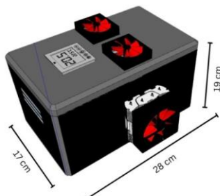
GAMBAR 2. Desain alat AWG TEC
