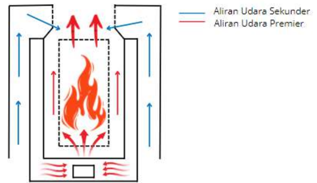
GAMBAR 3 (Skema aliran udara kompor biomassa)
