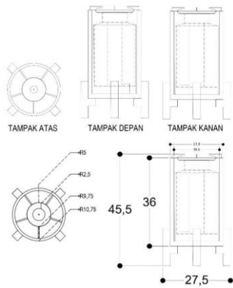
GAMBAR 1 (Desain Kompor 2D)
