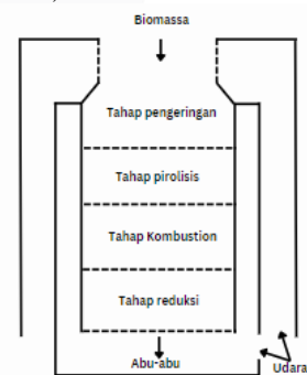
GAMBAR 4 (Skema Cara Kerja Kompor)
