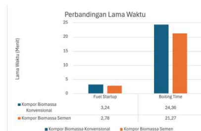
GAMBAR 2 (Grafik Perbandingan Lama Waktu)
