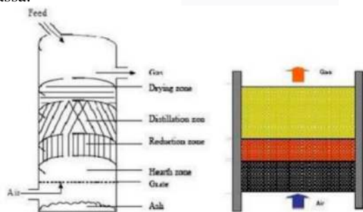
GAMBAR 1 (Skema Tungku Gasifikasi Updraft)
