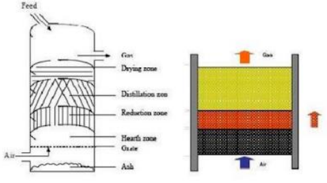
GAMBAR 1. Skema tungku gasifikasi updraft
