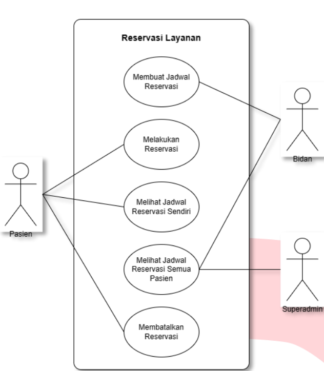
GAMBAR 2 Use Case Diagram Bagian Reservasi Layanan
