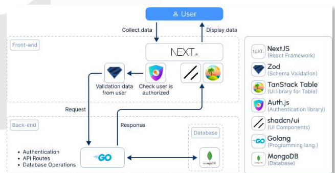
GAMBAR 1 Sistem Desain Aplikasi
