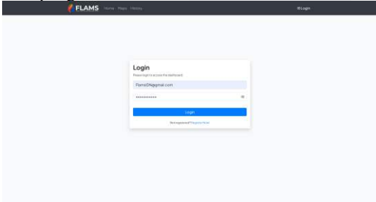
GAMBAR 11 Halaman Login
