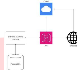
GAMBAR 1 Arsitektur Sistem
