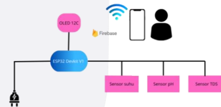
GAMBAR 3.2 Diagram blok rangkaian
