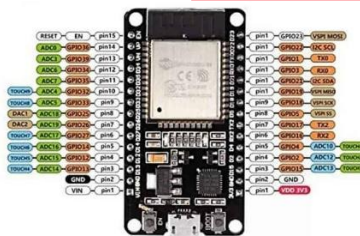
GAMBAR 2.2 ESP32 Devkit V1
