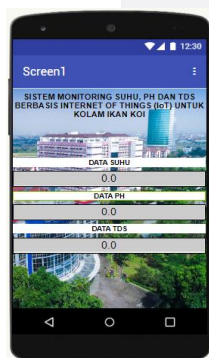
GAMBAR 3.4 Desain Aplikasi
