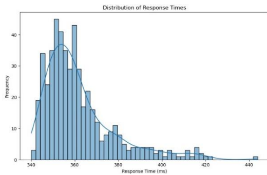
GAMBAR 7 Distribusi Waktu 500 User
