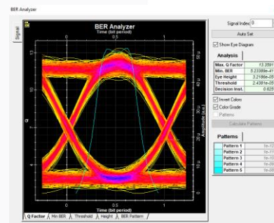
Gambar 14. Nilai BER dan Q-Factor XGPON Downstream
