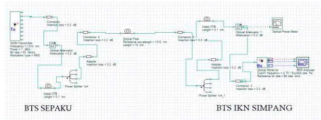
Gambar 10. Simulasi perancangan untuk NGPON disisi downlink
