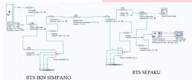
Gambar 11. Simulasi perancangan untuk XGPON dan NGPON disisi Uplink
