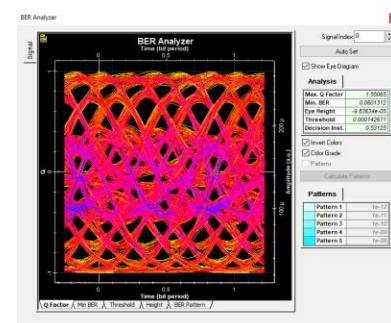
Gambar 15. Nilai BER dan Q-Factor NGPON Downstream
