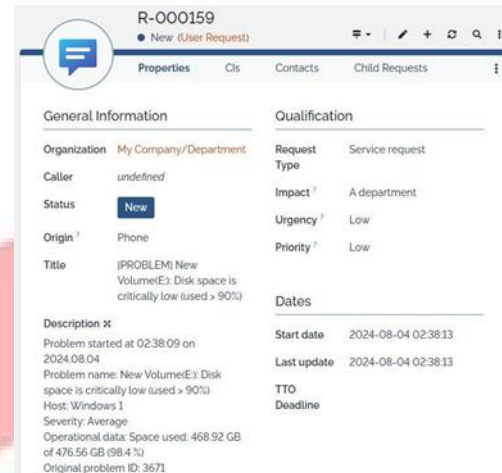
GAMBAR IV. 2 Tiket Helpdesk
