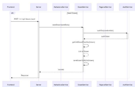
GAMBAR 10 Sinkronisasi Data Mahasiswa
