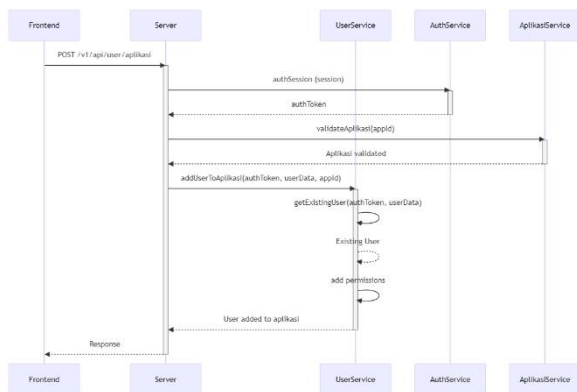
GAMBAR 11 Memberikan Akses Aplikasi Ke Pengguna
