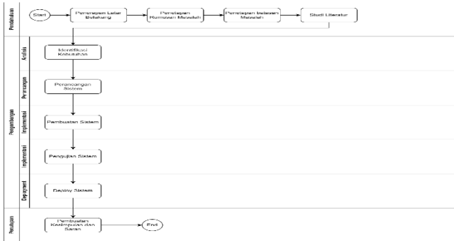
GAMBAR 4 Sistematika Penelitian
