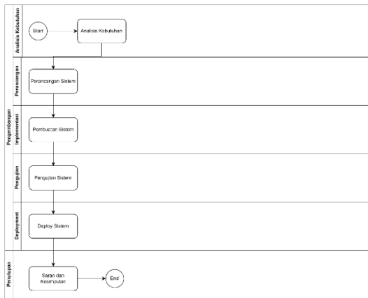
GAMBAR 3 Sistematika penelitian
