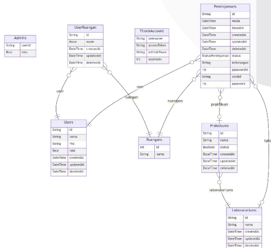
GAMBAR 14 ERD
