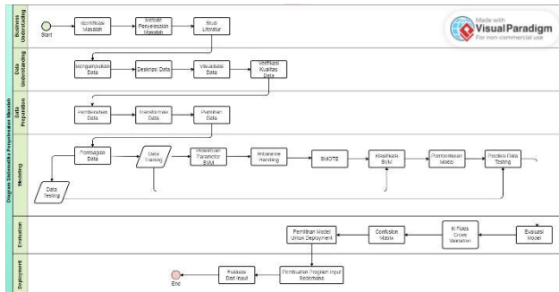
GAMBAR 4. Diagram Sistematika Penyelesaian Masalah
