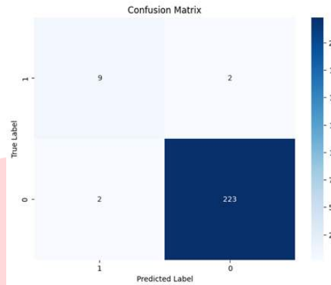
GAMBAR 7. Confusion Matrix Sebelum Smote
