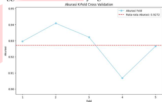
GAMBAR 10. K-Fold Cross Validation Setelah Smote
