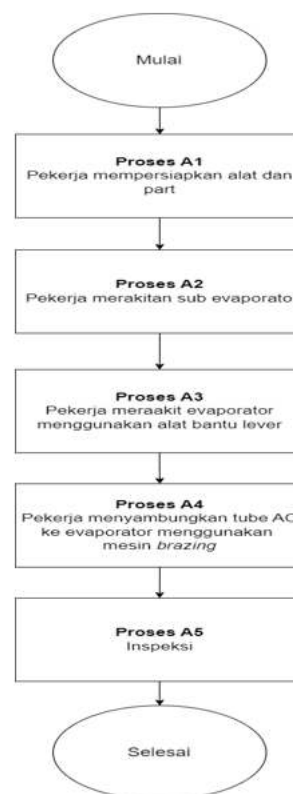
Gambar 1 Alur Proses Produksi Produk AC Mobil
