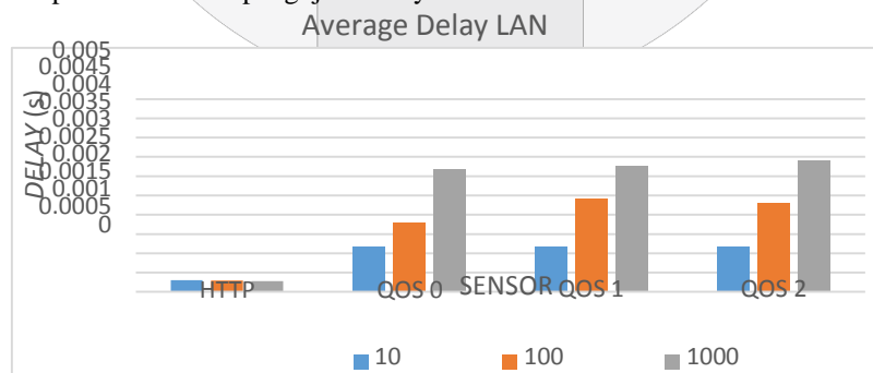
Gambar 4.1 Grafik Delay LAN
