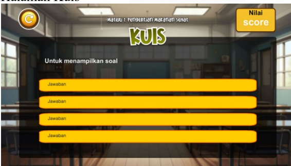
GAMBAR 5 (HALAMAN KUIS )
