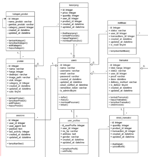
Gambar 4. Class Diagram Sistem UD Keluarga
