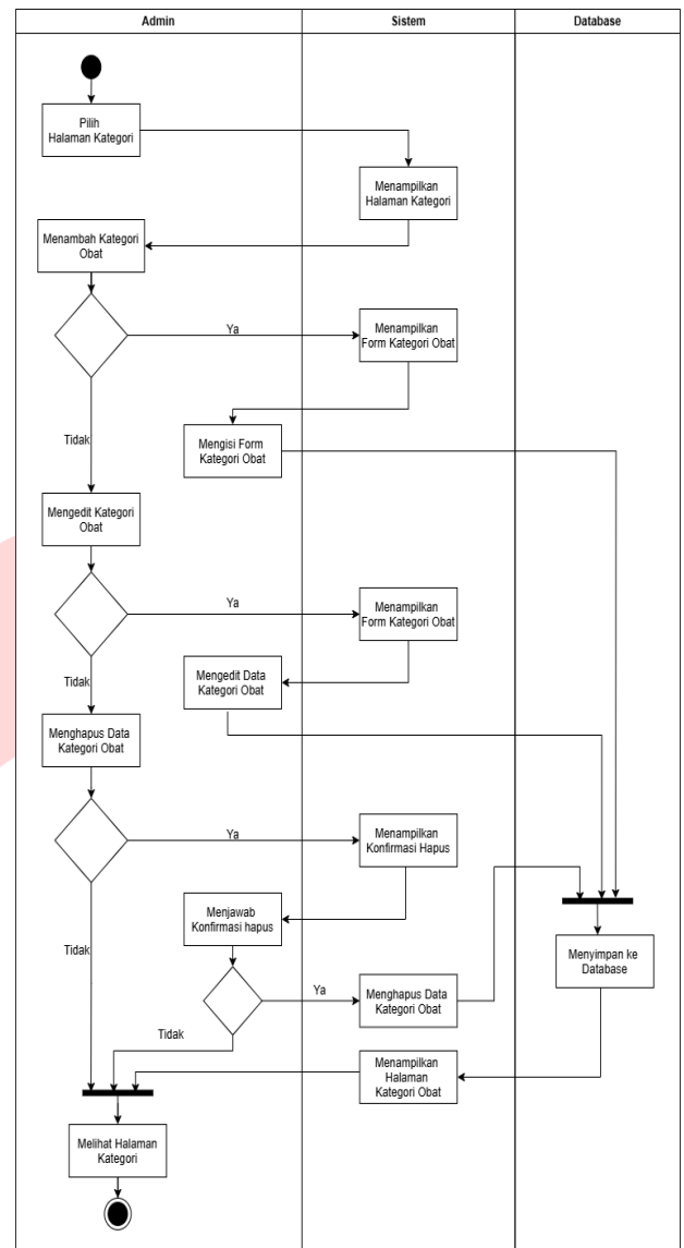
GAMBAR 9 (Activity Diagram Halaman Kategori Obat)
