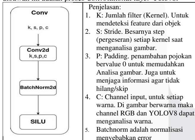
GAMBAR 2 (CONVOLUTION LAYER YOLOV8)
