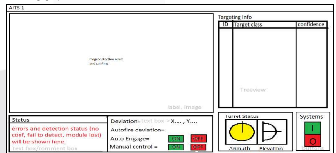
GAMBAR 11 (CONTOH LAYOUT GUI YANG DIRENCANAKAN)
