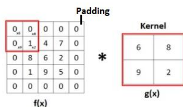
GAMBAR 3 KERNEL DAN PADDING DI SISTEM CNN
