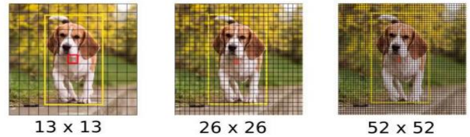
GAMBAR 4 (ILUSTRASI PEMBAGIAN CONVOLUTION LAYER YOLO UNTUK DETEKSI OBJEK)
