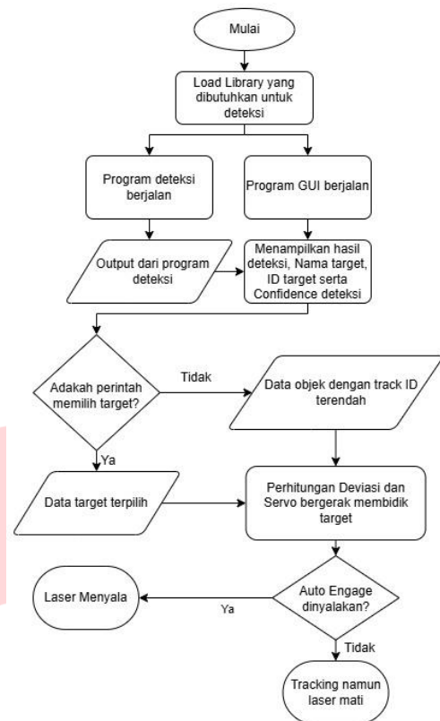
GAMBAR 10 (FLOWCHART CARA KERJA SISTEM DETEKSI DAN GUI TURRET)
