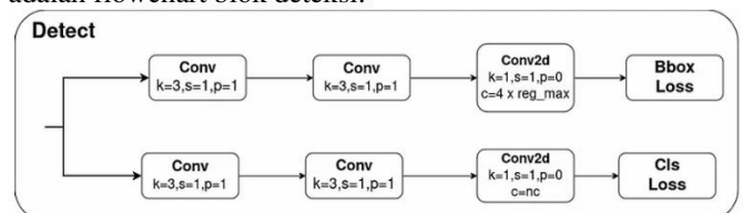
GAMBAR 1 (FLOWCHART BLOK DETEKSI)
