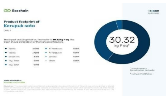
GAMBAR 1. 2 EUTROFICATION
