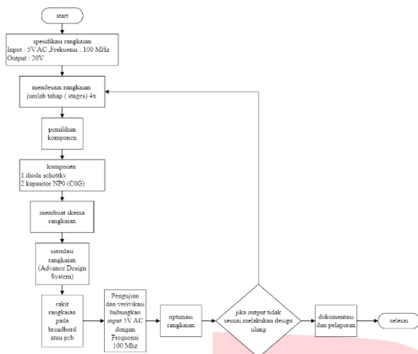
GAMBAR 7 (FLOWCHART Pengerjaan)
