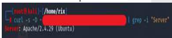
GAMBAR 12 (INFORMASI SERVER TERLIHAT PADA HEADER)
