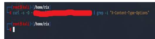
GAMBAR 13 (INFORMASI SERVER TERLIHAT PADA HEADER)
