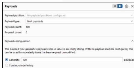
GAMBAR 5 (MENGATUR PAYLOAD)
