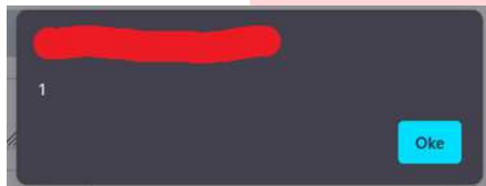
GAMBAR 4 (XSS BERHASIL)
