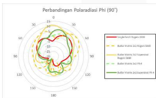
GAMBAR 10 Perbandingan Hasil Pola Radiasi
