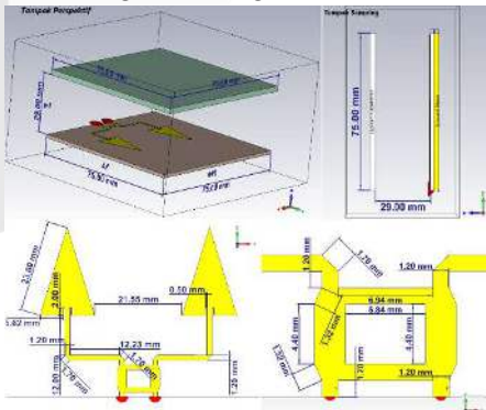
GAMBAR 7 Antena Butler Matrix 2x2 Dengan Lapisan Superstrat Menggunakan Rogers 5880.
