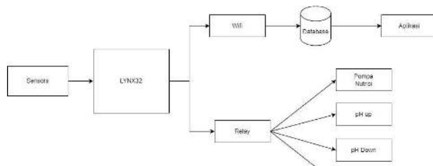
GAMBAR 5 Blok Diagram Otomatisasi
