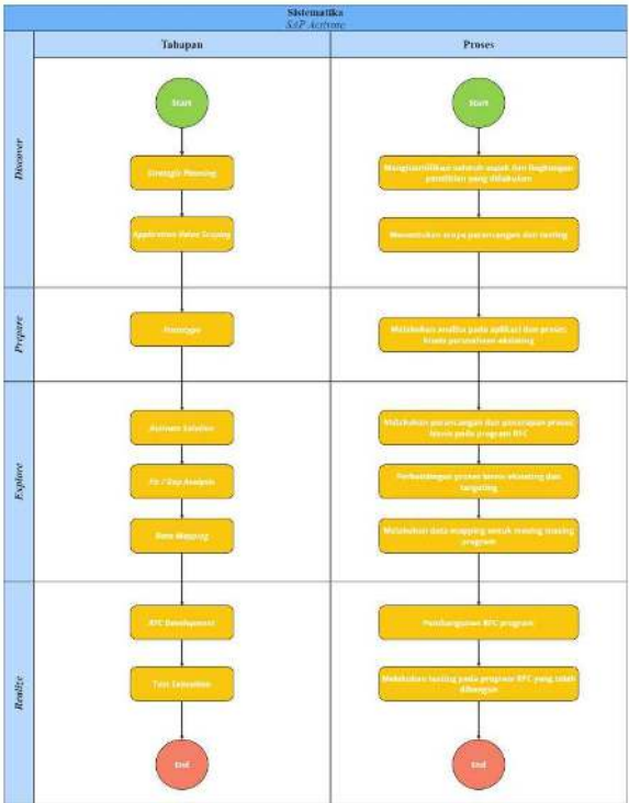
GAMBAR 3 (Metodologi SAP Activate)
