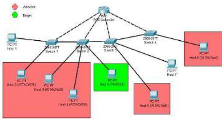
GAMBAR 2 Topologi SDN
